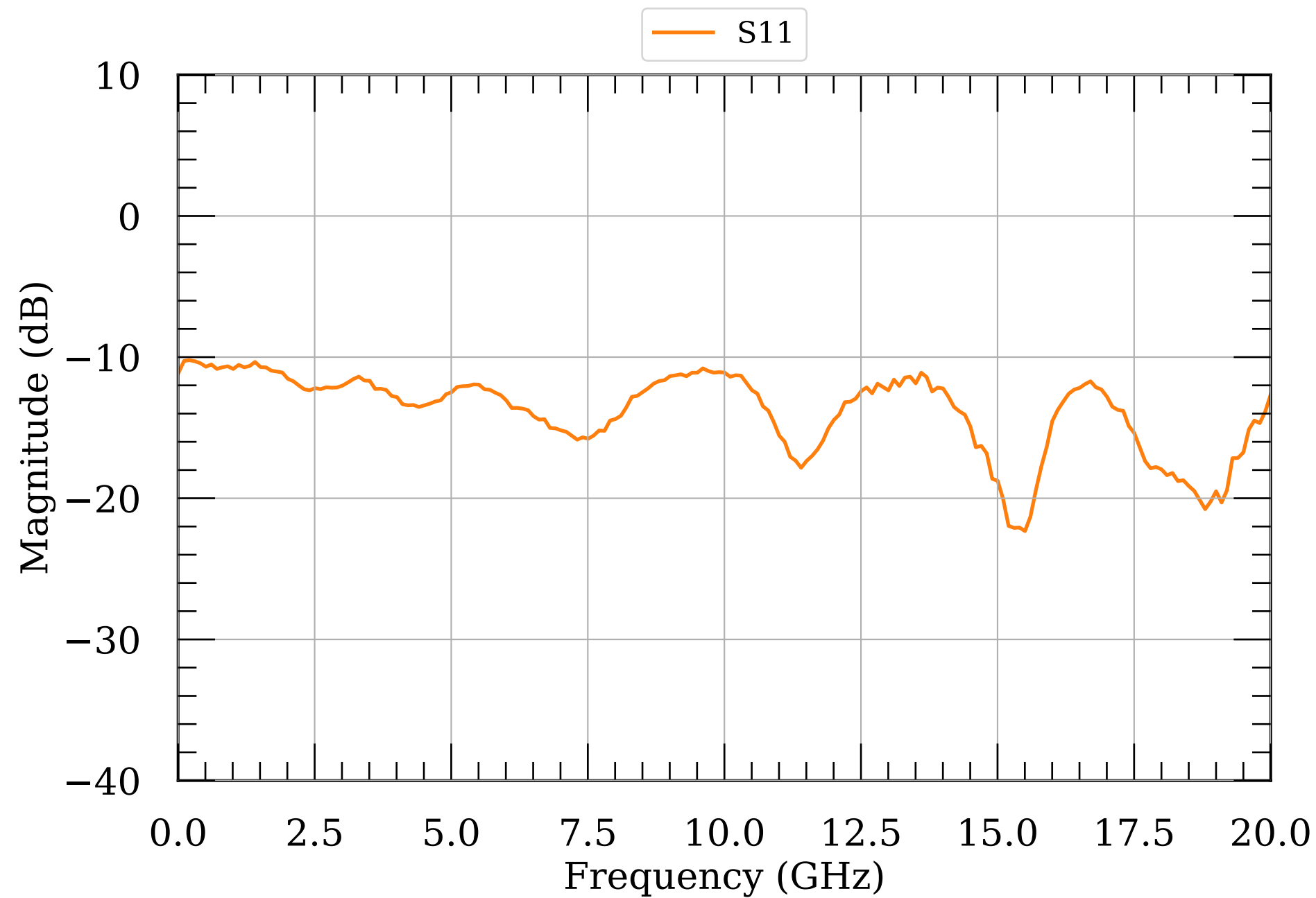
LNA S-params module072
